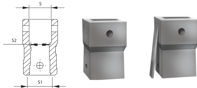
Vana mili adaptörü / Spindle Adaptor
